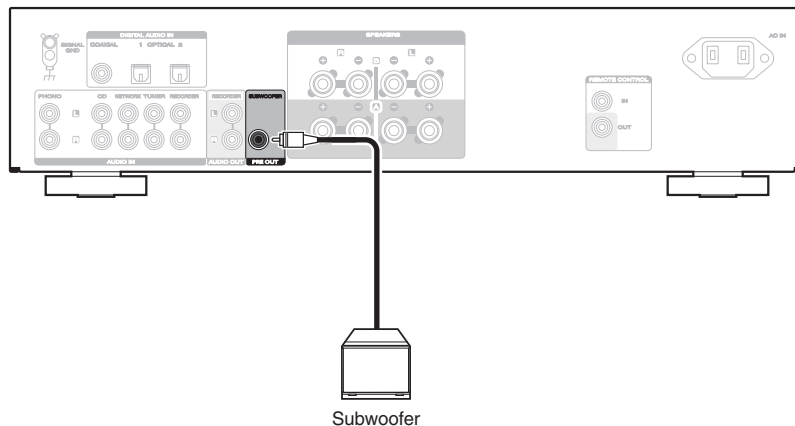
Subwoofer
