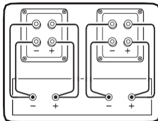
Bi-cablare
