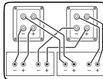
Conexiune Bi-Amping
